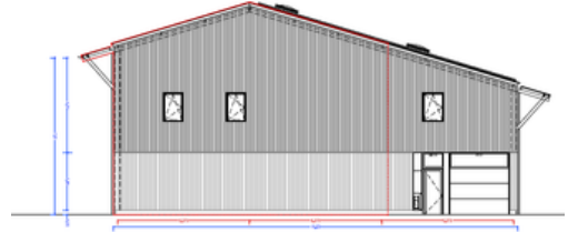
FACADE SUD-EST
